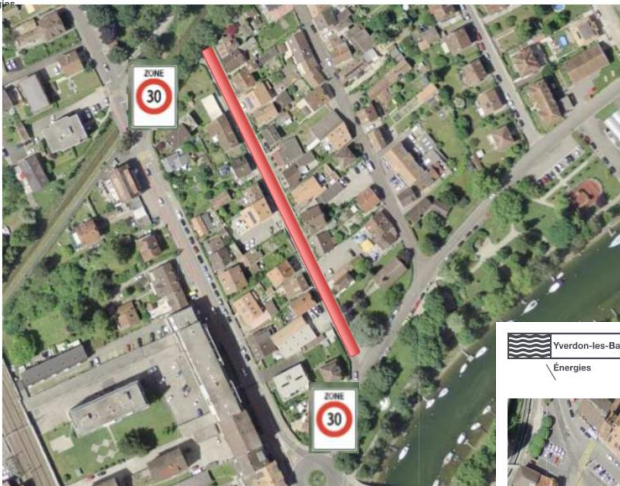
Zone d'intervention renouvellement des réseaux
